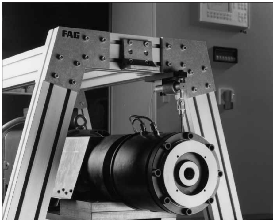
Banco de ensayos FE8 de FAG
