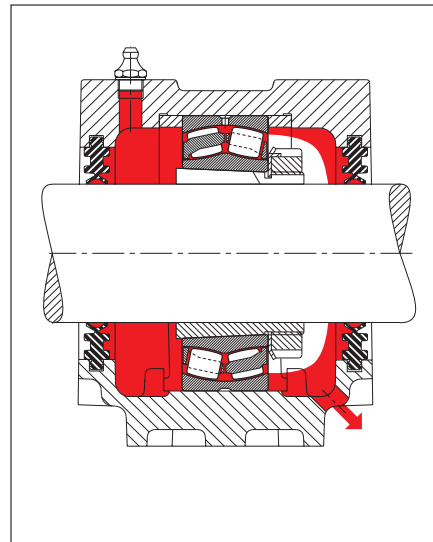
43: Relubricación con grasa. El engrase excesivo se evita mediante un orificio de evacuación
