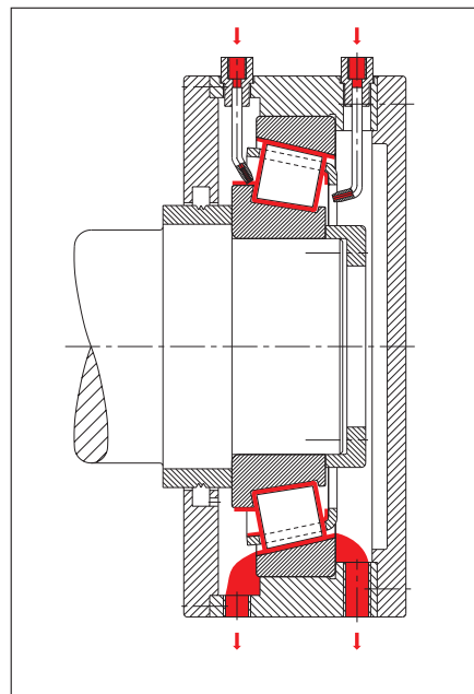
63: Alimentación de aceite por ambos lados en rodamientos de rodillos cónicos
